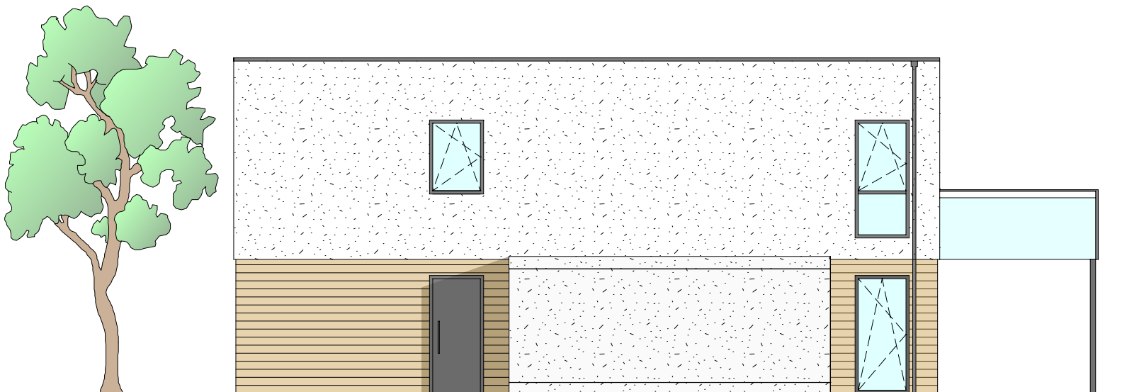
Südwest-Ansicht
